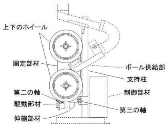
【各部の名称を示す参考右側面図】
