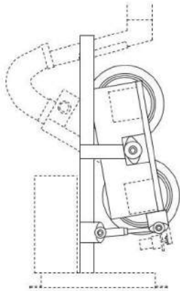
【第二の傾斜状態を示す参考左側面図】
