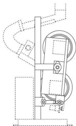
【第一の傾斜状態を示す参考左側面図】
