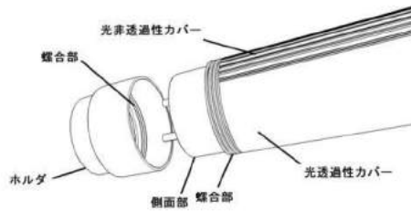
【分解参考斜視図】
