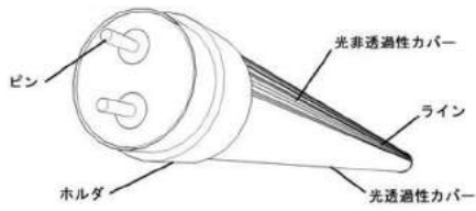
【使用状態及び各部の名称を示す参考斜視図】
