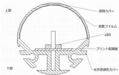
【各部の名称を示す参考断面図】
