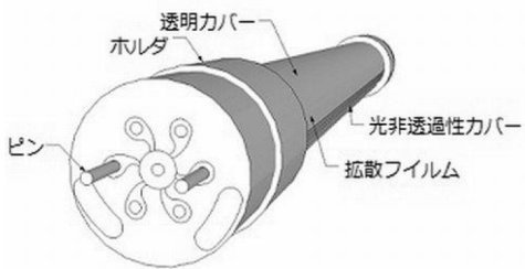
【使用状態及び各部の名称を示す参考図】
